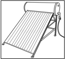
Solar water panels (sólár guáter pánel) Paneles solares de agua
